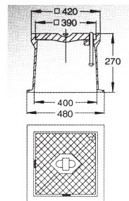
Unterflurdeckel quadratisch
