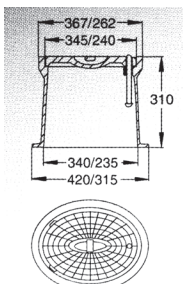
Unterflurdeckel oval
