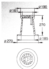
Unterflurdeckel rund
